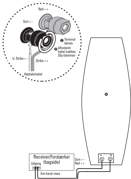
Figur 3. Tegning viser kabeltilslutning med korrekt polaritet for een kanal i et surroundsystem.
